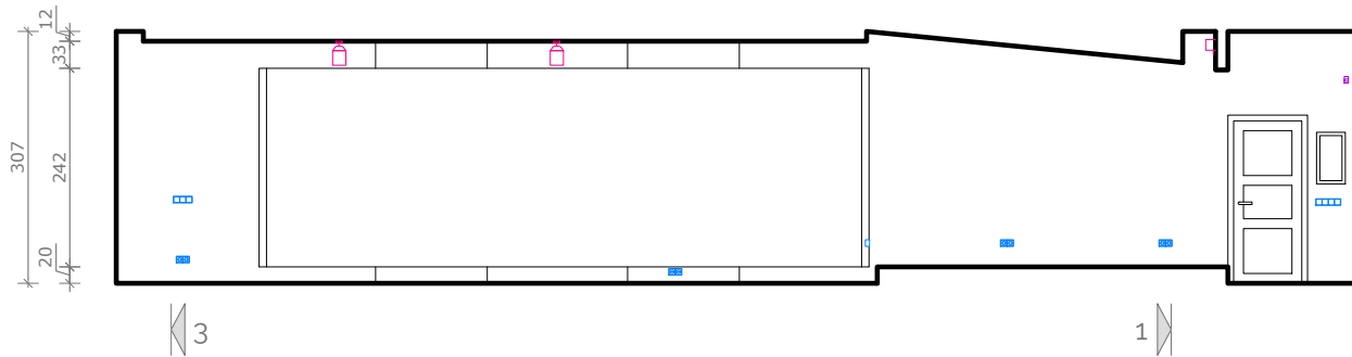
Išklotinė 4
